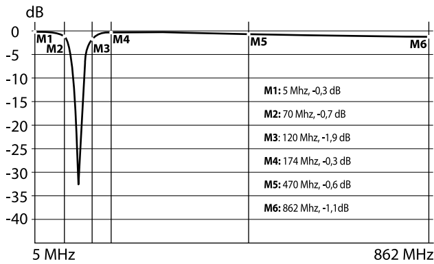
Coupling attenuation IN→TV
